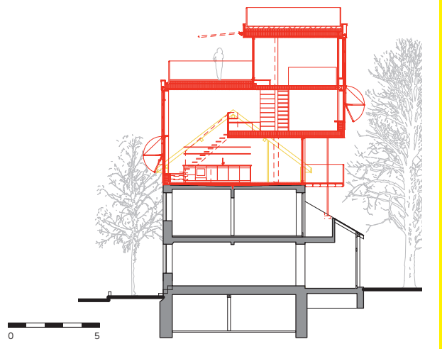
Schnitt
